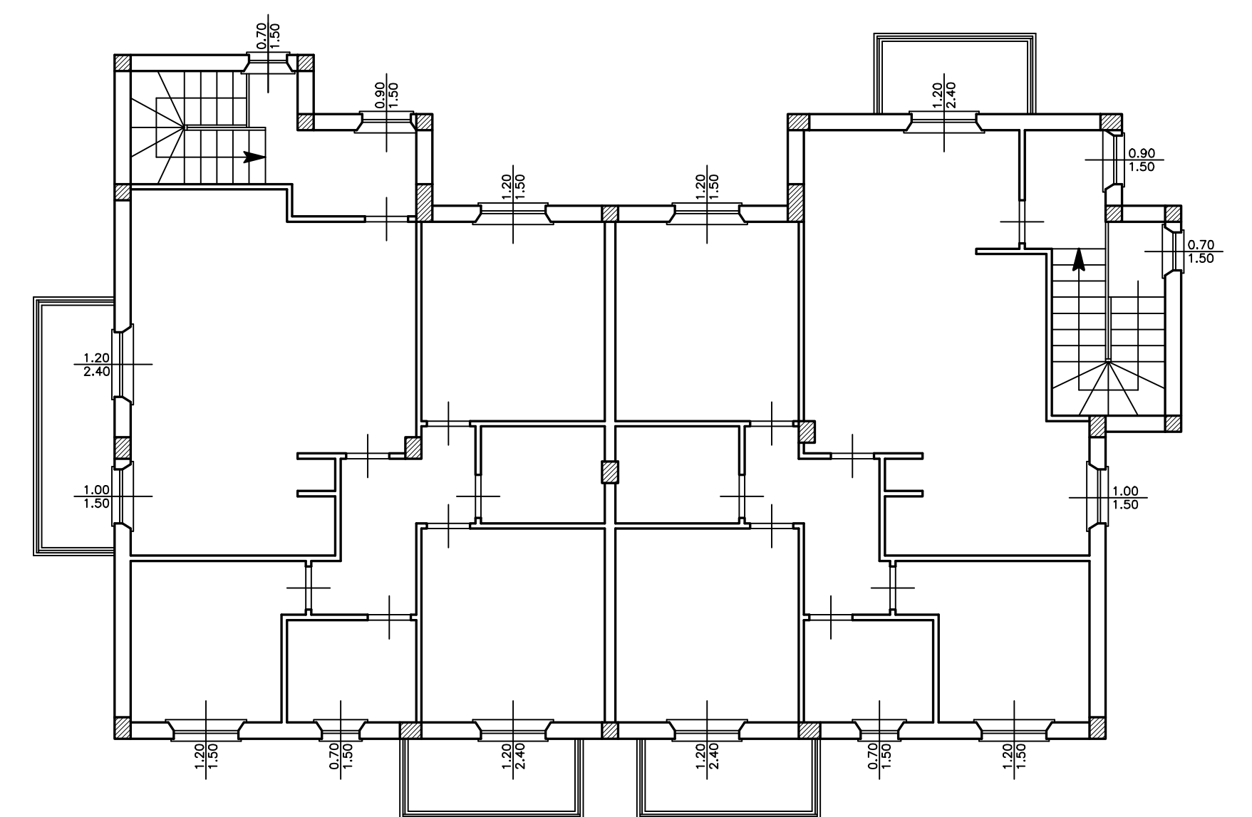
PIANO PRIMO
